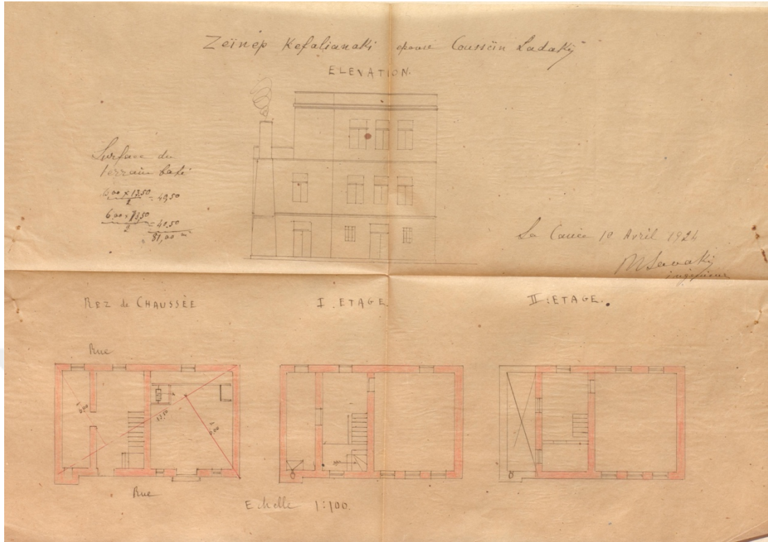
Resim 3.7.: Mehmet Kefalyanaki'nin kızı Zeynep Hanım'ın tasfiye talepnamesinde bulunan ev krokisi 168
